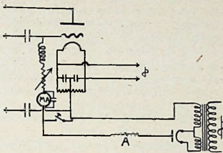
Fig. 3. Bij den blokkeeringscondensator links beneden den mA-meter schrijve men de aanduiding C'.
