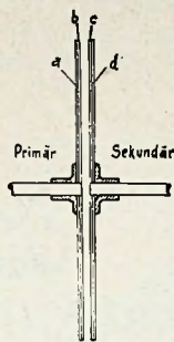
Fig. 5. Doorsnede door de 4 schijven; de primaire schijven a en b, waarvan a vast met de as is verbonden, doch b niet met de as, doch na instelling met a; voorts de secundaire schijven met radiale spleten, waarvan weer c vast met een as is verbonden en d niet met de as, doch met c.
