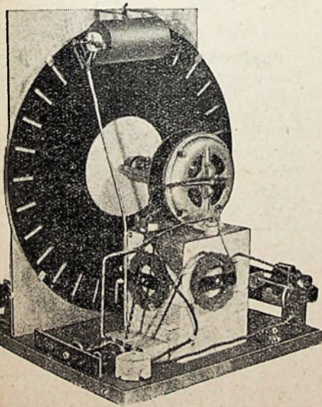
De eerste universele „Arnei“-televisie-ontvanger (systeem Fries). Achterzijde.
