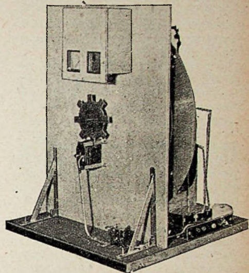
De eerste universele „Arnei“-televisie-ontvanger (systeem Fries). Voorzijde.
