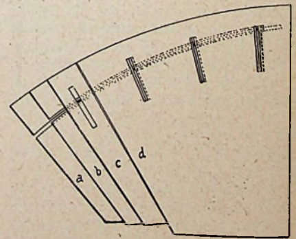
Fig. 4. Twee schijven met spiraalspleet volgens fig. 1 (a en b) en twee schijven met radicale spleten volgens fig. 2 (c en d) over elkaar gelegd; a en c zijn elk met een as verbonden; b is draaibaar om de as van a en d draaibaar om de as van c; na instelling kan b met a vast verbonden worden, evenals d met c. Men ziet, hoe door het op elkaar leggen der ten opzichte van elkaar verschoven schijven de grootte der gaatjes kan worden gewijzigd.
