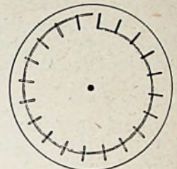
Fig. 3. De schijf met spiraalspleet en die met radicale spleten over elkaar gelegd. Bij doorkijk ontstaan sectorvormige gaatjes evenals bij de normale Nipkow'sche schijf.
